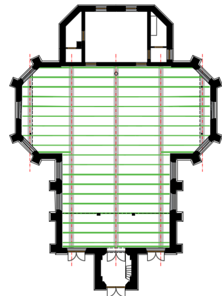
VLOERENPLAN
